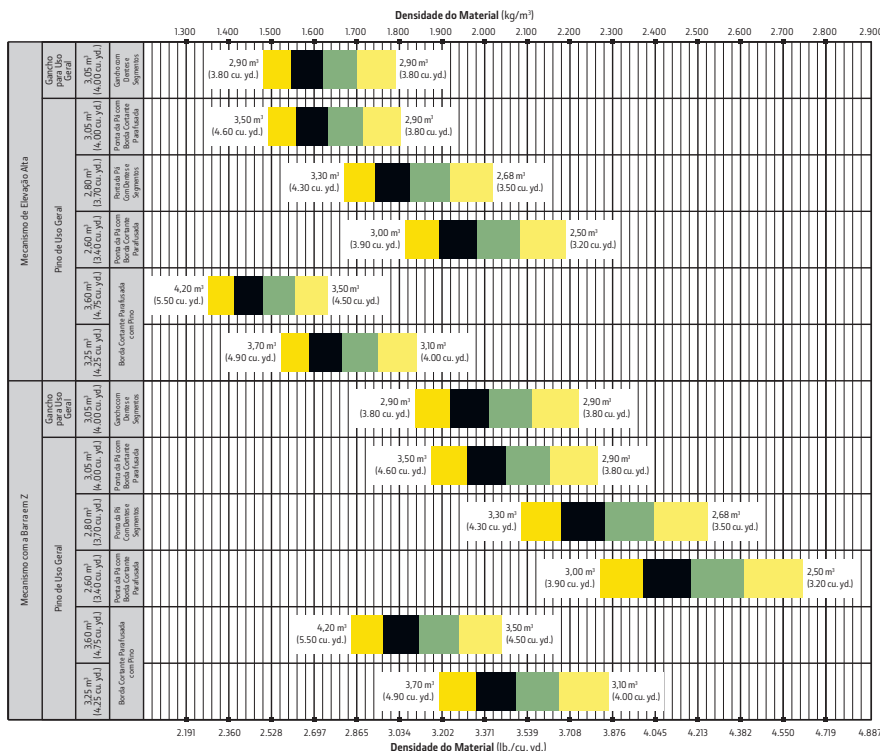
Fatores de Enchimento da Caçamba
